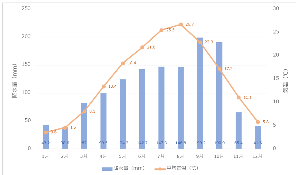
気象観測点(久喜)における平年値(統計期間 1991～2020 年)
