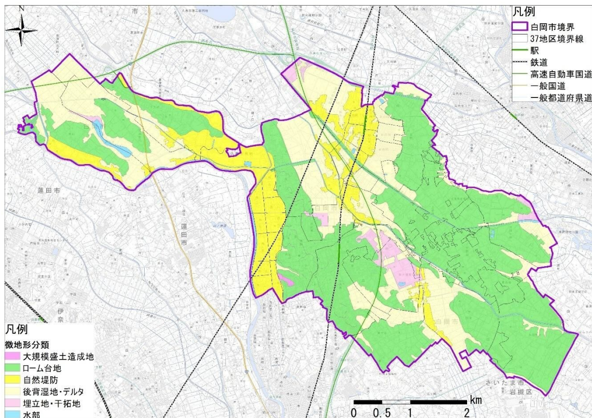
白岡市の地形分類図
